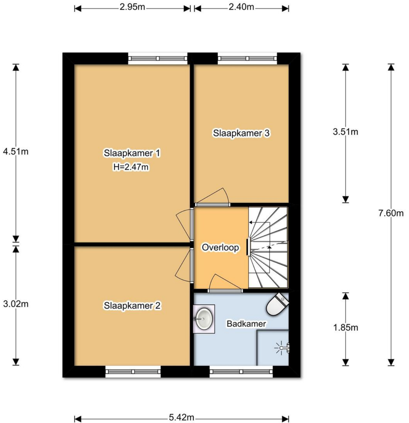
1e Verdieping
