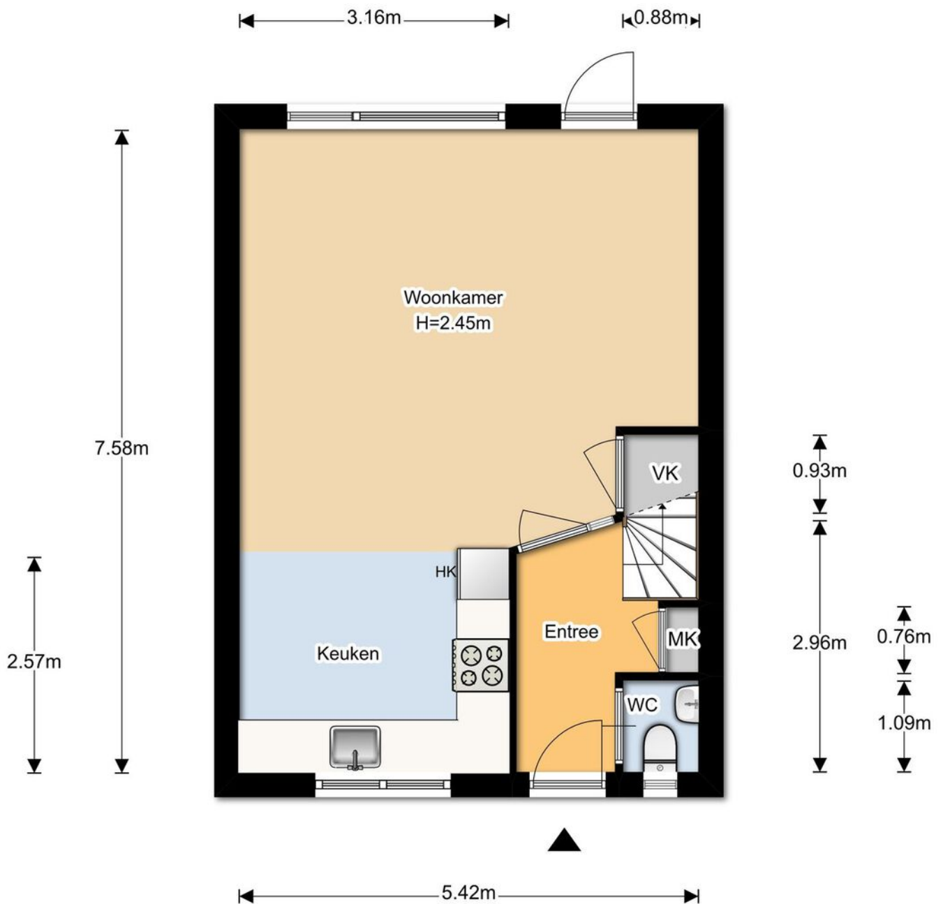
Begane Grond
